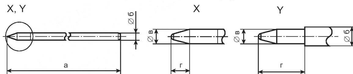
Рисунок 2 — Типы стержней D, E и F
