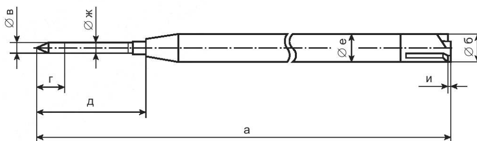
Рисунок 4 — Тип стержня G 2
