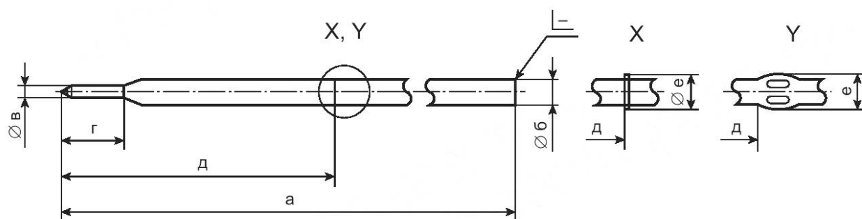
Рисунок 1 — Типы стержней A 1 , A 2 и B
