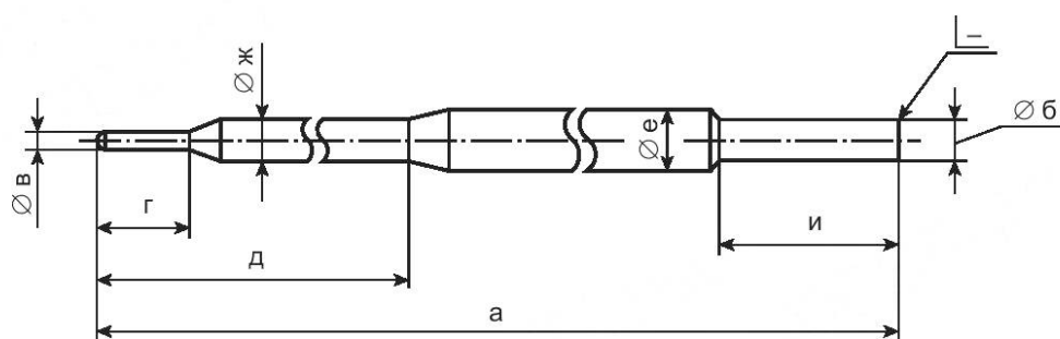
Рисунок 3 — Тип стержня G 1
