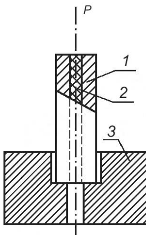
1 — оболочка карандаша; 2 — стержень; 3 — подставка
