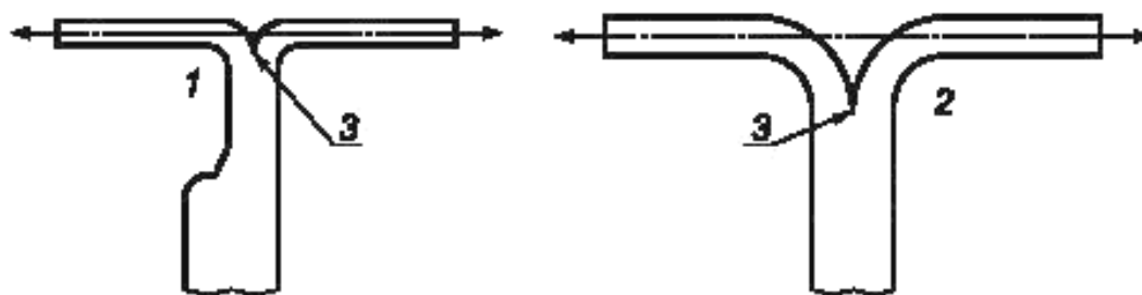
Рисунок 1 — Положение линии разделения слоев
