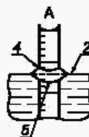
1 — жидкость; 2 — горизонтальная плоская поверхность жидкости; 3 — нижняя часть мениска; 4 — место считывания шкалы; 5 — мениск
