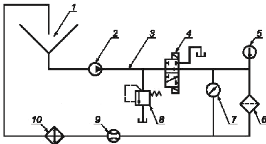
1 — введение загрязнителя; 2 — насос; 3 — другой вариант места введения загрязнителя; 4 — распределитель электрогидравлический; 5 — датчик температуры; 6 — испытываемый фильтроэлемент; 7 — дифференциальный манометр; 8 — клапан предохранительный; 9 — расходомер; 10 — теплообменник
