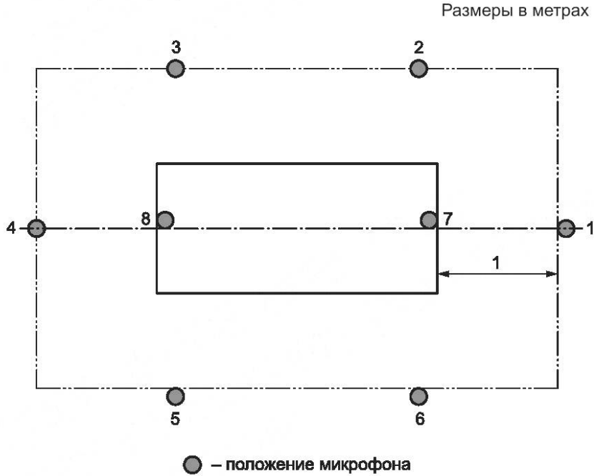
Рисунок D.3 — Вид сверху на машину (показана огибающим параллелепипедом)
