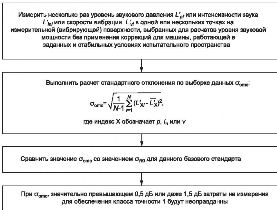
Рисунок С.1 — Блок-схема процедуры оценки \sigma_{omc} с рекомендацией по выбору соответствующего базового стандарта
