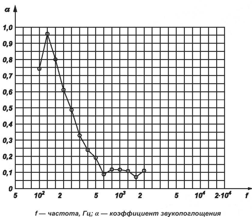
Рисунок В.2 — Коэффициент звукопоглощения для мембранного звукопоглотителя в реверберационном помещении объемом 200 м 3
