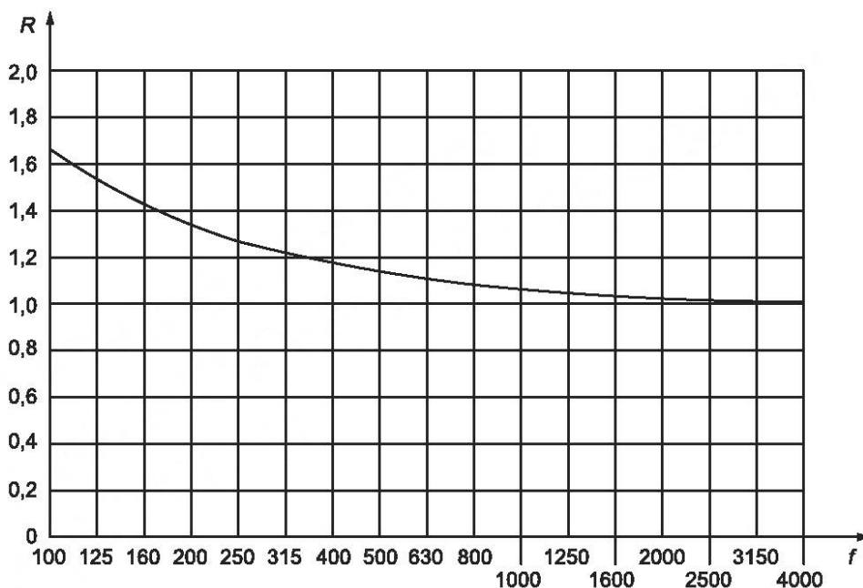
Рисунок 1 — График зависимости реверберационного параметра R от частоты для камеры объемом 70 м³
