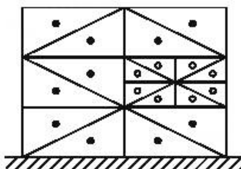
Рисунок С.6 — Пример дополнительных точек измерений на части измерительной поверхности в виде параллелепипеда с разбиением на треугольные участки
