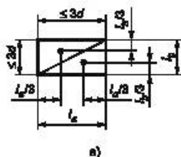
Рисунок С.4 — Основные точки установки микрофонов на измерительной поверхности в виде параллелепипеда с разбиением на треугольные участки
