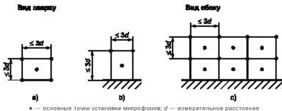
Рисунок С.1 — Основные точки установки микрофонов на измерительной поверхности в виде параллелепипеда с разбиением на прямоугольные участки
