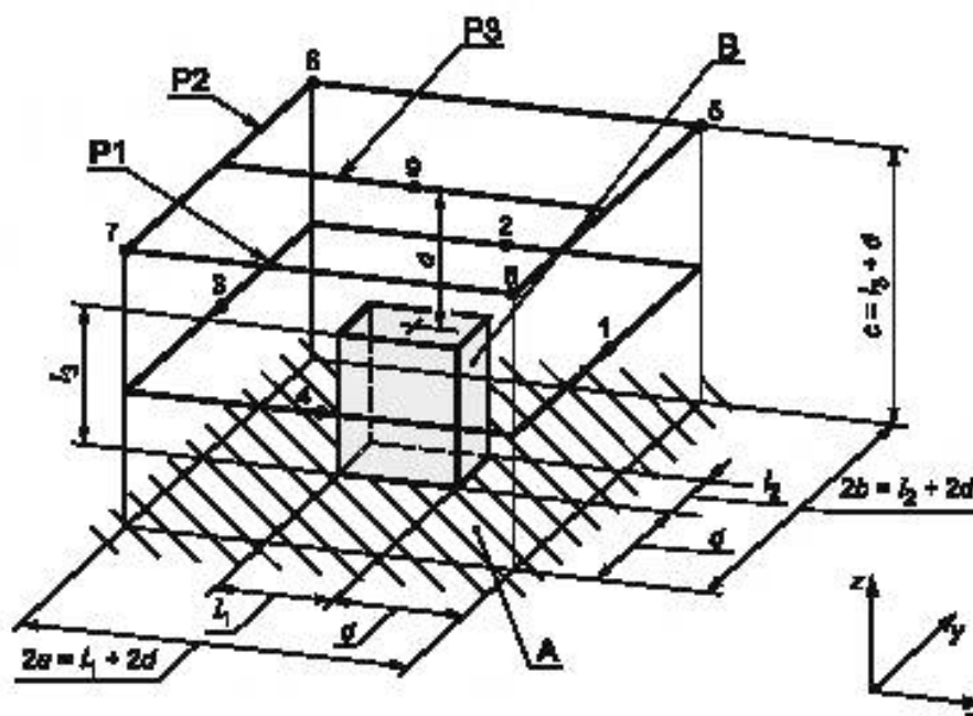
Рисунок С.6 — Пример дополнительных точек измерений на части измерительной поверхности в виде параллелепипеда с разбиением на треугольные участки
