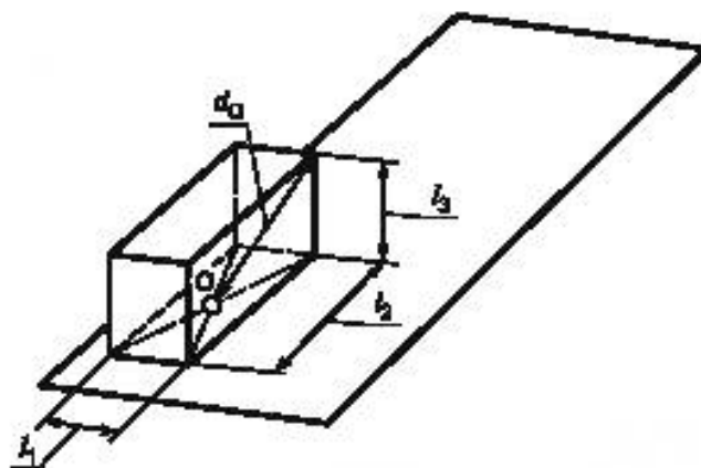
а) Одна звукоотражающая плоскость, d_0 = \sqrt{(l_1/2)^2 + (l_2/2)^2 + l_3^2}
