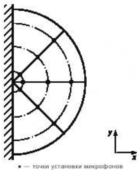
Рисунок D.3 — Пример расположения микрофонов на верхнем основании измерительной поверхности в виде половины цилиндра в случае двух звукоотражающих плоскостей
