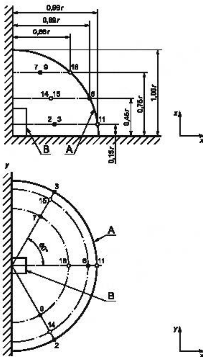
Рисунок В.3 — Точки установки микрофонов на полусферической измерительной поверхности в случае двух звукоотражающих плоскостей
