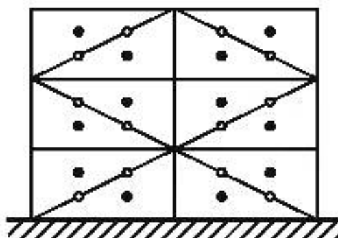
Рисунок С.5 — Дополнительные точки установки микрофонов по всей измерительной поверхности в виде параллелепипеда с разбиением на треугольные участки
