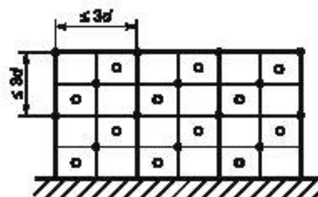
Рисунок С.2 — Дополнительные точки установки микрофонов по всей измерительной поверхности в виде параллелепипеда с разбиением на прямоугольные участки
