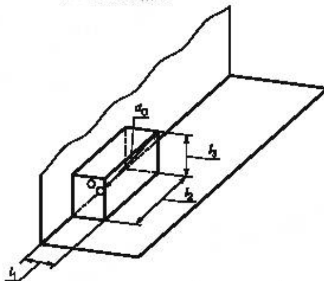
б) Две звукоотражающие плоскости, d_0 = \sqrt{l_1^2 + (l_2/2)^2 + l_3^2}
