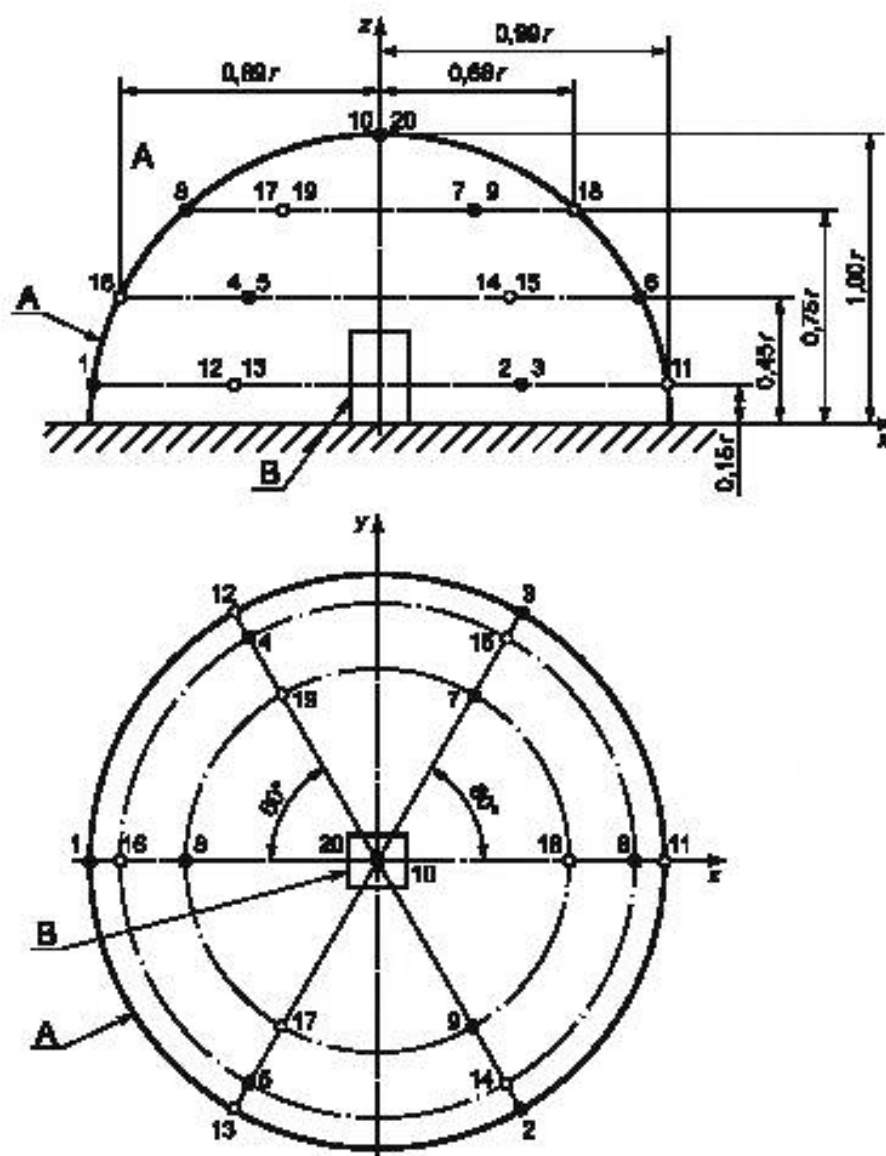
Рисунок В.2 — Точки установки микрофонов на полусферической измерительной поверхности для испытаний источников широкополосного шума
