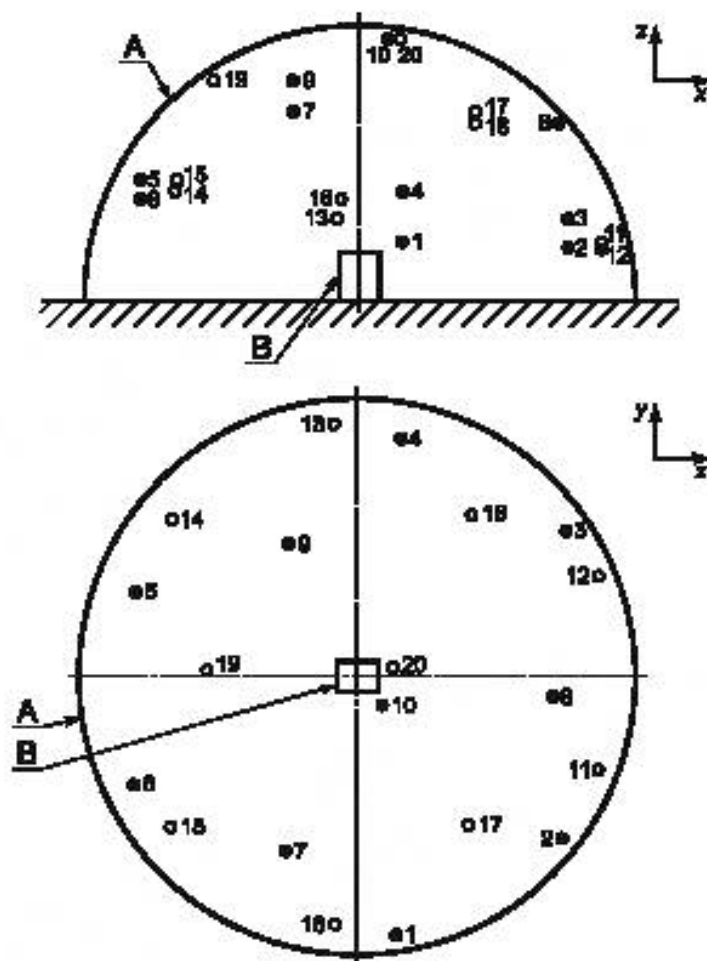
Рисунок В.1 — Предпочтительные точки установки микрофонов на полусферической измерительной поверхности для испытаний источников шума всех видов
