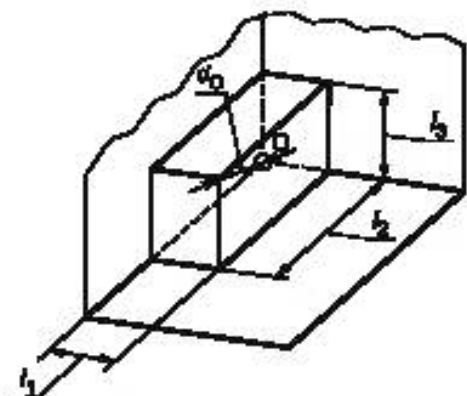
с) Три звукоотражающие плоскости, d_0 = \sqrt{l_1^2 + l_2^2 + l_3^2}
