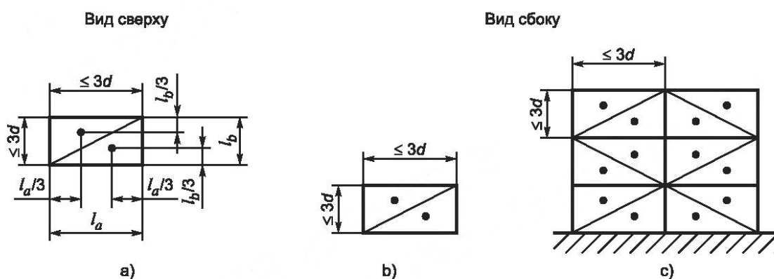
Рисунок С.3 — Пример дополнительных точек измерений на части измерительной поверхности в виде параллелепипеда с разбиением на прямоугольные области
