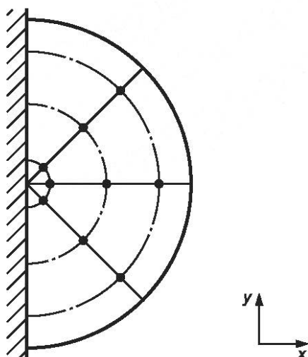
Рисунок D.2 — Пример расположения микрофонов в случае пяти траекторий сканирования на боковой поверхности и четырех на верхнем основании
