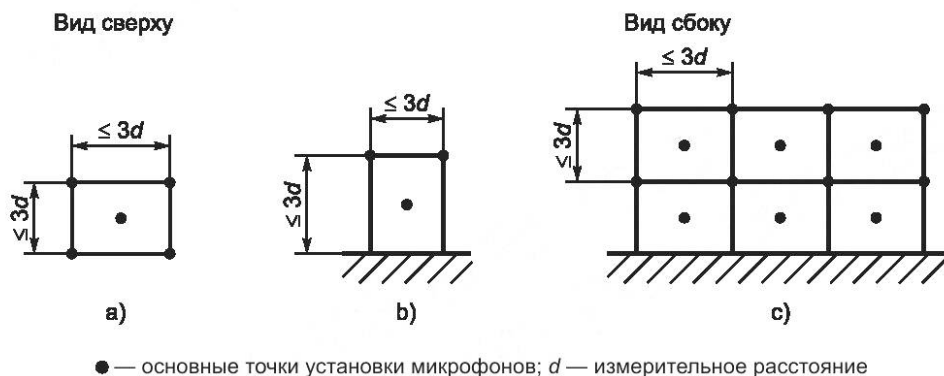
Рисунок С.1 — Основные точки установки микрофонов на измерительной поверхности в виде параллелепипеда с разбиением на прямоугольные области
