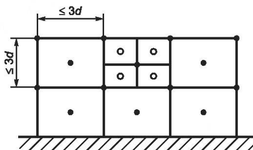
Рисунок С.2 — Дополнительные точки установки микрофонов по всей измерительной поверхности в виде параллелепипеда с разбиением на прямоугольные области
