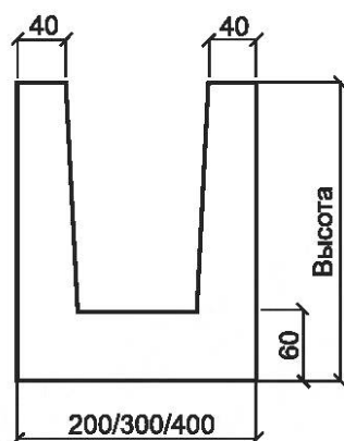
б) Сечение
