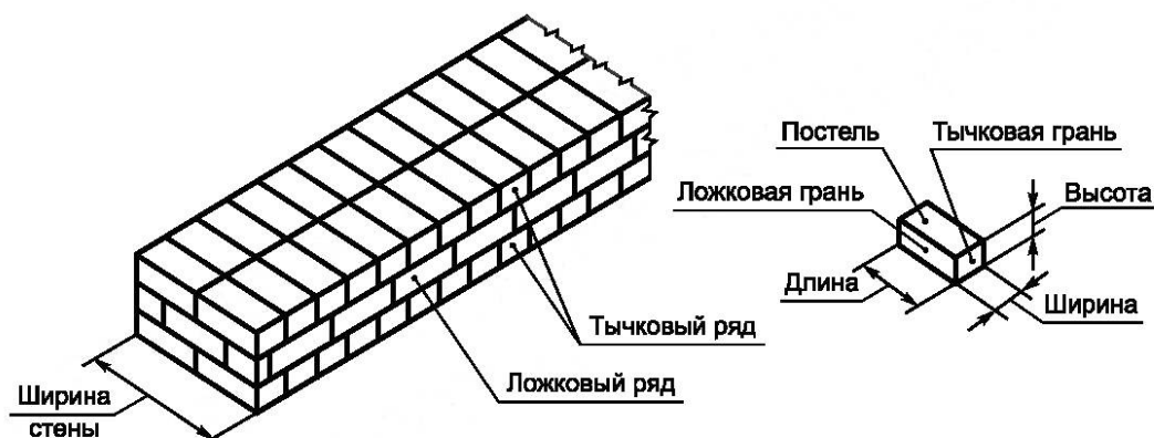
Рисунок 1 — Кирпичная кладка
