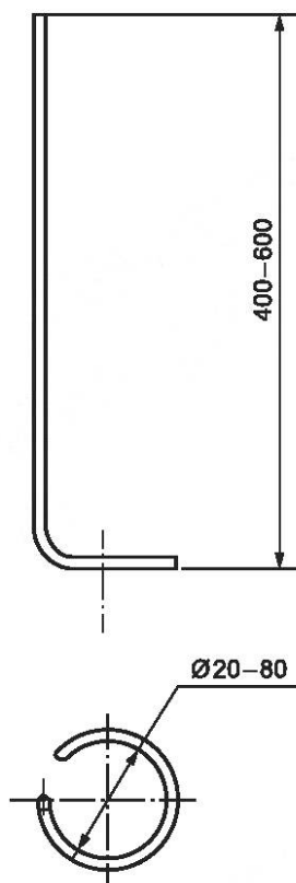
Рисунок 1 — Мешалка
