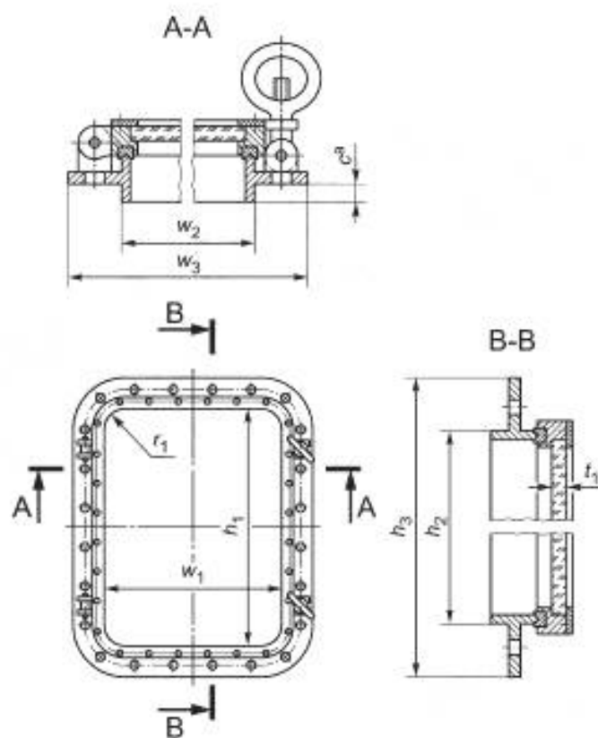
а) Способ крепления окна – болтами
