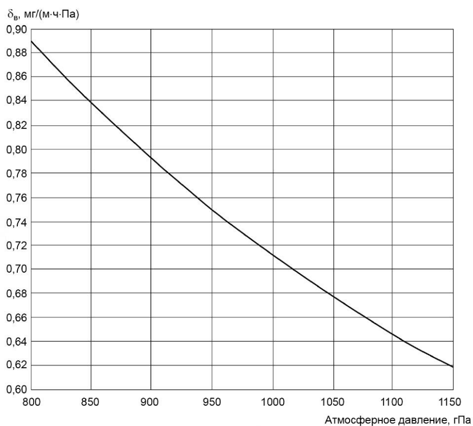
Рисунок Б.1 — Паропрооницаемость воздуха при температуре 23 °C
