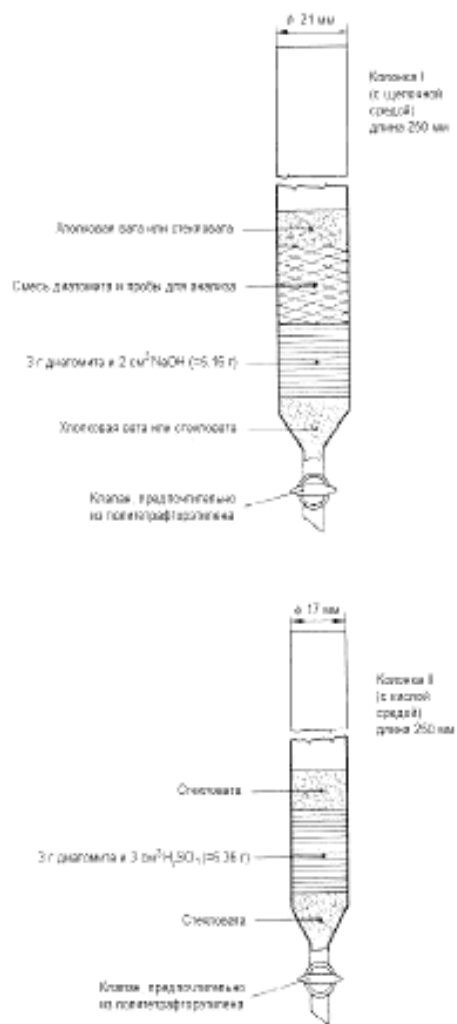
Рисунок 1 – Хроматографические колонки
