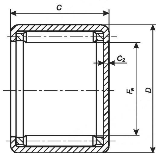
Рисунок 7 — Конструктивное исполнение ВК
