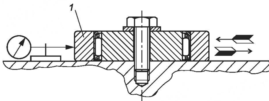
1 — калибр-кольцо
