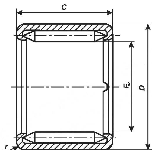
Рисунок 3 — Конструктивные исполнения НК и 09
