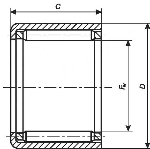
Рисунок 8 — Конструктивное исполнение ГК
