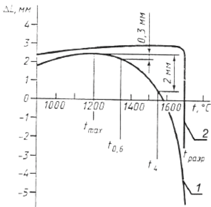
1 – для алюмосиликатных огнеупоров; 2 – для периклазовых огнеупоров.
