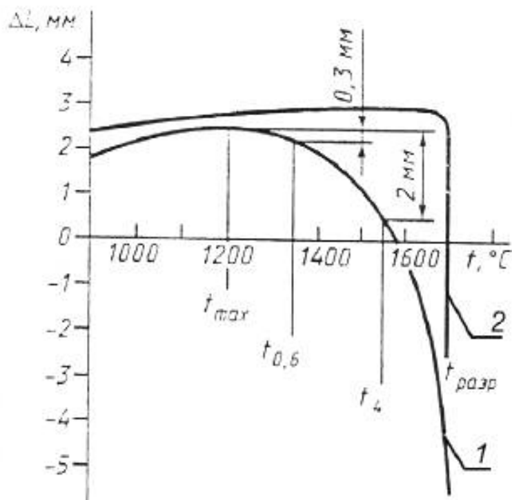
1 — для алюмосиликатных огнеупоров; 2 — для периклазовых огнеупоров.
