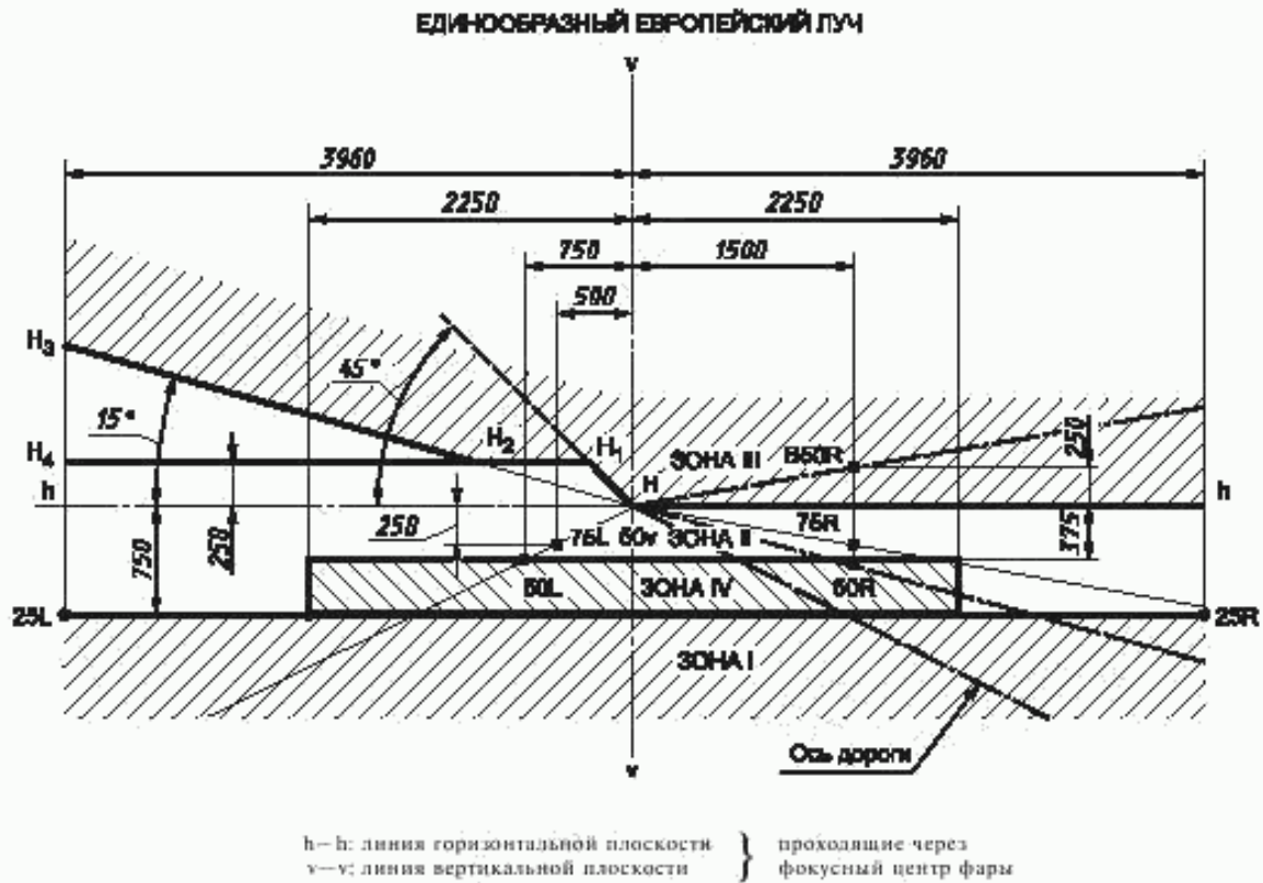
Рисунок В — Фара для левостороннего движения
