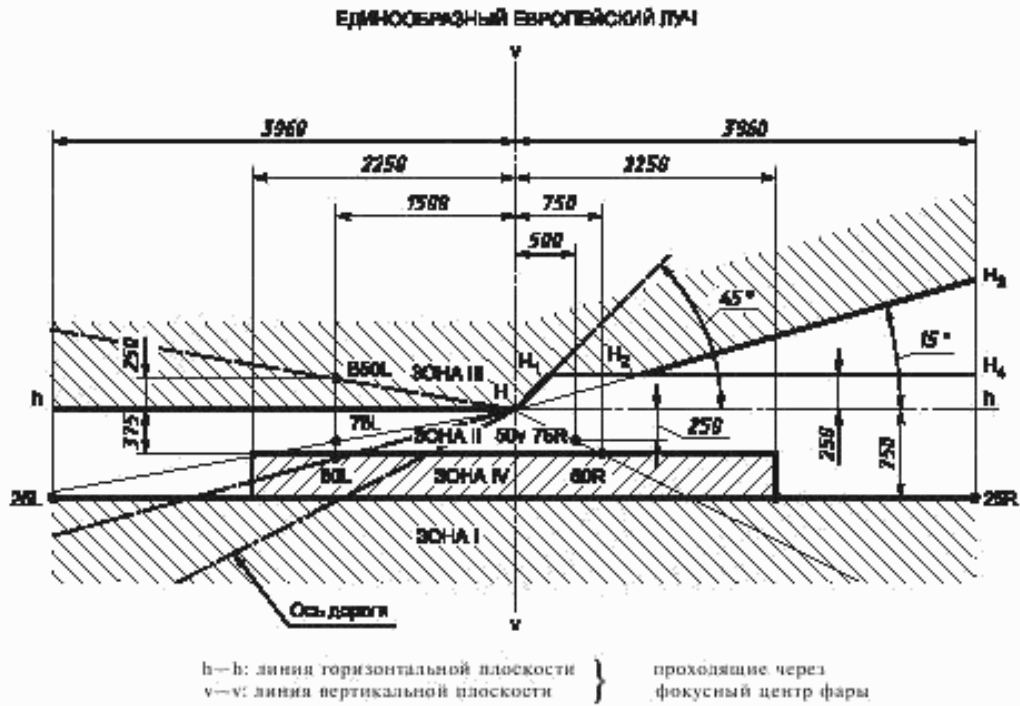
Рисунок А — Фара для правостороннего движения
