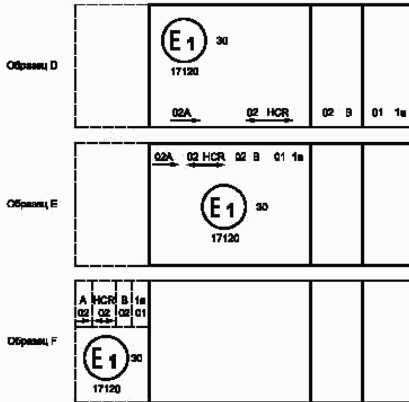
6 Совмещенная фара
