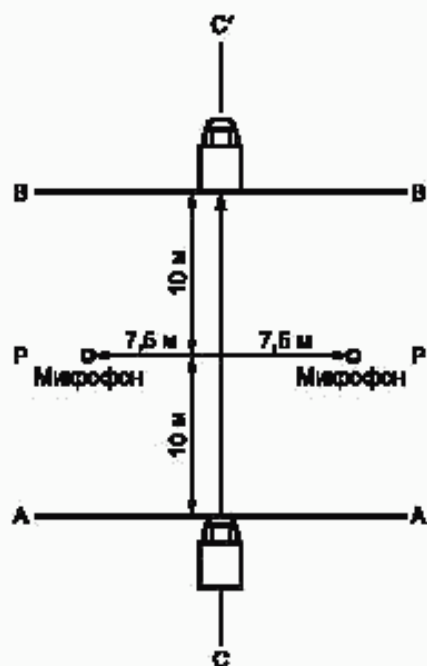
Рисунок 3.1 — Положения движущихся транспортных средств при измерениях
