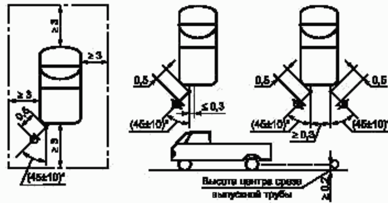
Рисунок 3.2 — Положения неподвижных транспортных средств при измерениях
