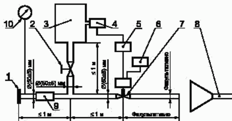
1 — впускной фланец или патрубок для подсоединения к задней части испытуемой системы выпуска; 2 — регулирующий клапан с ручным управлением; 3 — компенсационная емкость с максимальным объемом 40 л, время заполнения которой составляет не менее 1 с; 4 — реле давления с рабочим интервалом 0,05—2,5 бар; 5 — переключатель с задержкой по времени; 6 — счетчик импульсов; 7 — клапан быстрого действия, аналогичный заслонке газодинамического тормоза, диаметром 60 мм, приводимый в действие пневматическим цилиндром с выходным усилием 120 Н при давлении 4 бар. Время срабатывания как при открытии, так и при закрытии не должно превышать 0,5 с; 8 — отвод отработавших газов; 9 — гибкий патрубок; 10 — манометр
