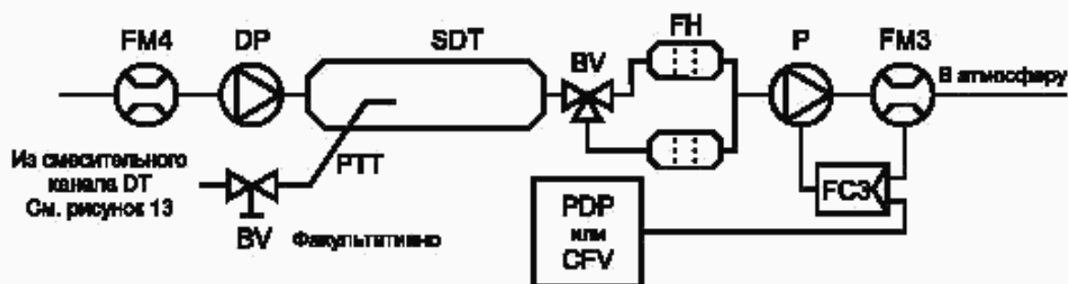
Рисунок 15 — Система разрежения (только система полного потока)
