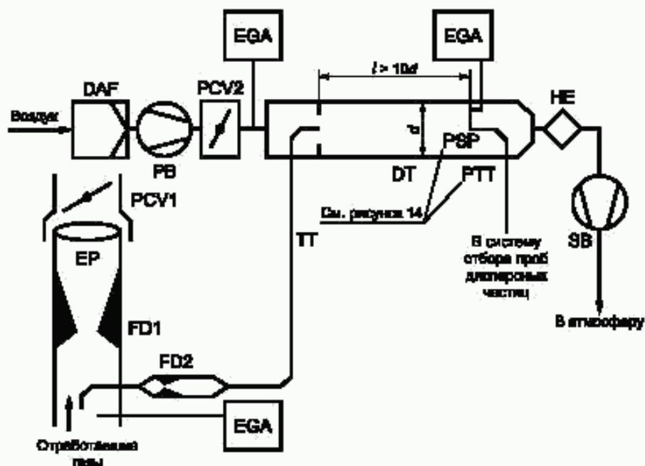
Рисунок 9 — Система разрезания части потока с двойной трубкой Вентури или двойным диафрагмовым расходомером, измерением концентрации \text{CO}_2 или \text{NO}_x и частичным отбором проб
