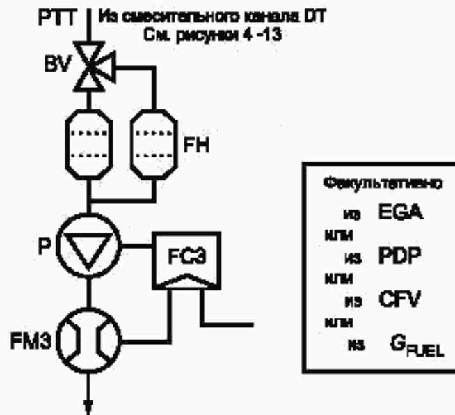
Рисунок 14 — Система отбора проб дисперсных частиц
