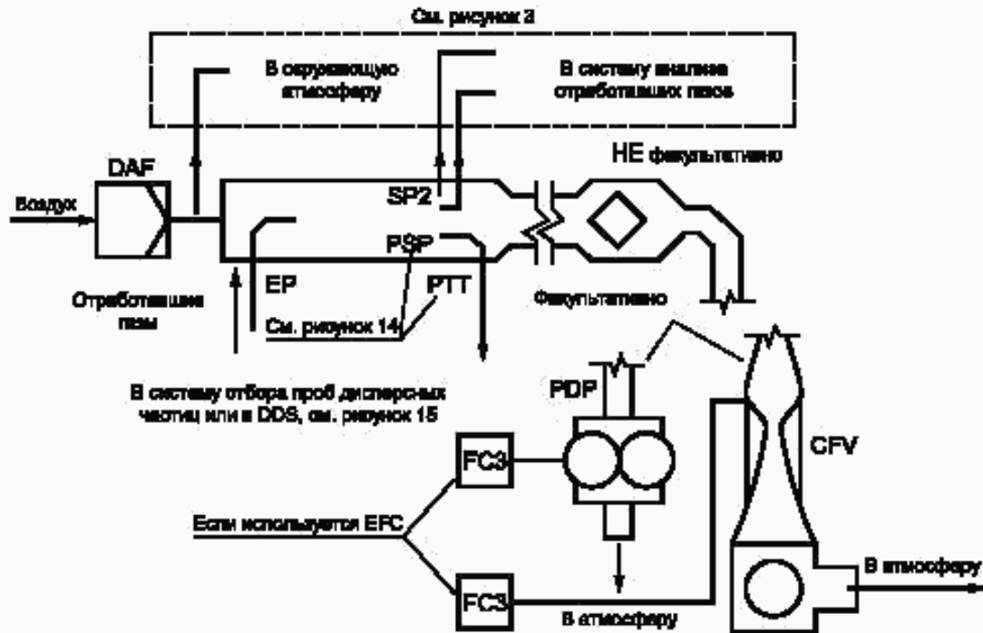
Рисунок 13 — Система разрежения полного потока
