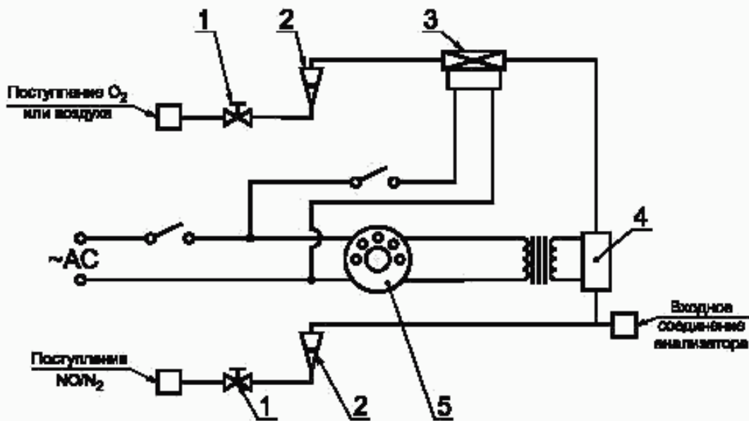
1 — клапан управления расходом; 2 — расходомер; 3 — электромагнитный клапан управления расходом; 4 — озонатор; 5 — вариатор
