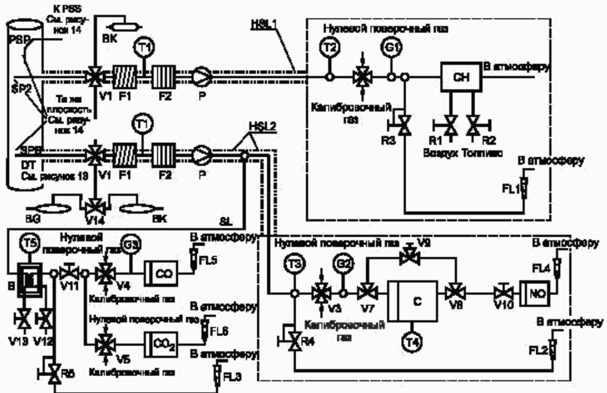
Рисунок 3 — Принципиальная схема системы анализа разреженных отработавших газов для измерения содержания \text{CO} , \text{CO}_2 , \text{NO}_x и \text{CH}
