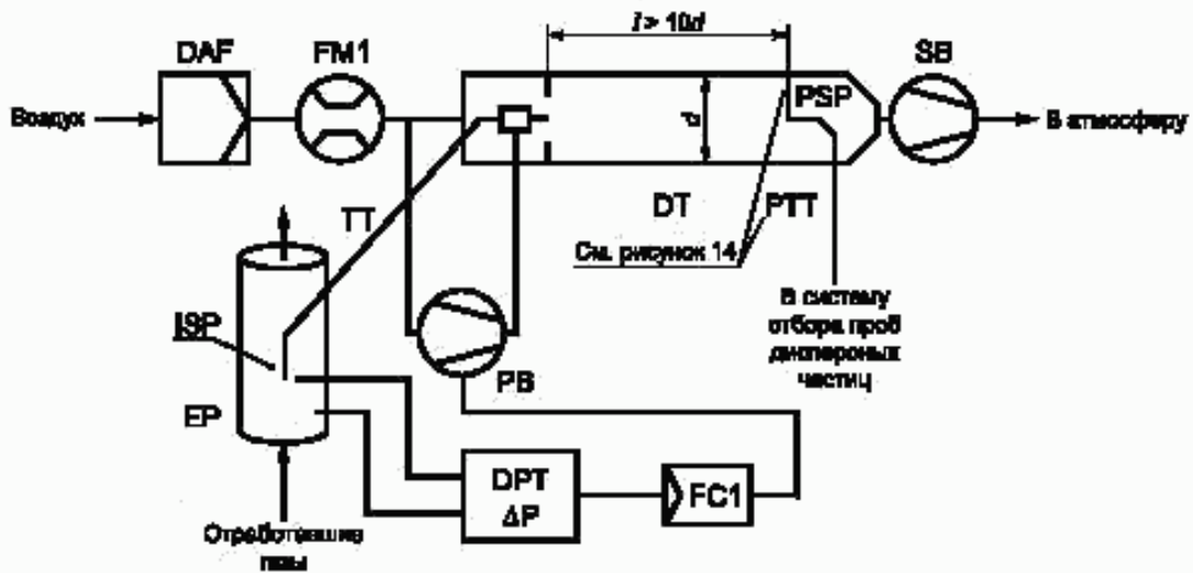
Рисунок 5 — Система разведения части потока с изокинетическим пробоотборником и частичным отбором проб (контроль PB)
