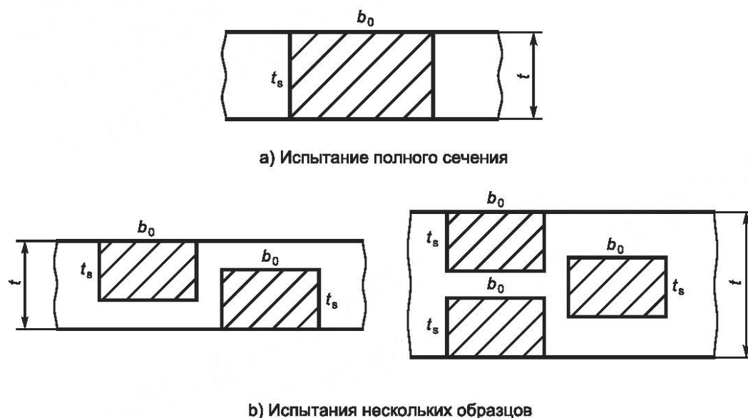
Рисунок 1 — Примеры расположения образцов для испытаний в соединениях
