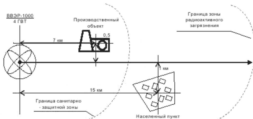
Рисунок Б.1 – Схема расположения производственного объекта относительно объекта использования атомной энергии
