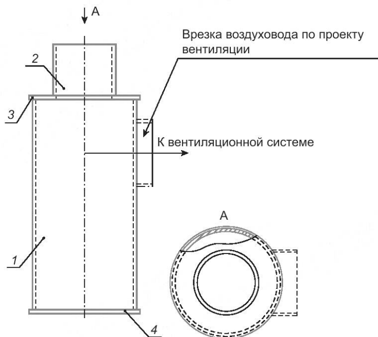
Рисунок А.1 — Схема конструктивного исполнения РК при присоединении воздухопроводов сбоку
