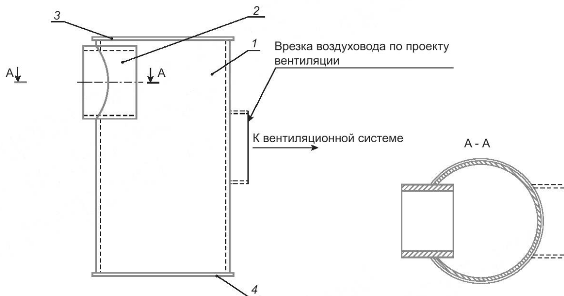
Рисунок А.1 — Схема конструктивного исполнения РК при присоединении воздухопроводов сбоку
