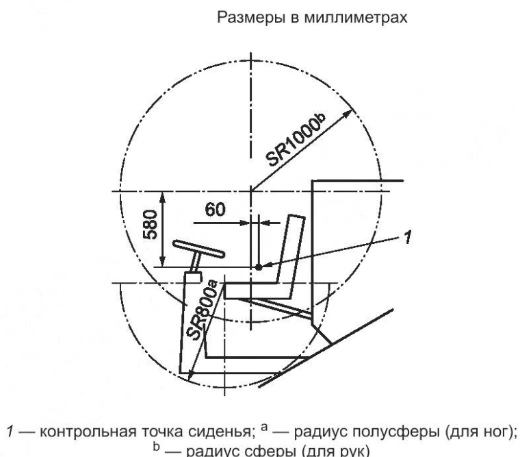
Рисунок 1 — Зона досягаємості рук і ног оператора
