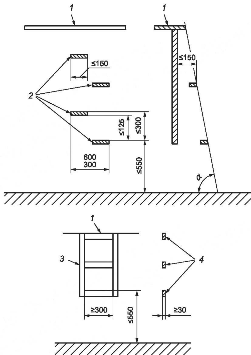
1 — платформа; 2 — ступень; 3 — лестница; 4 — ступень
