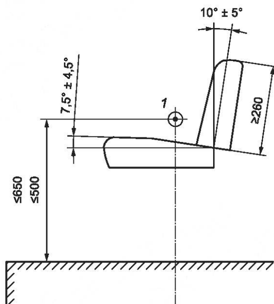
а) среднее положение регулировки сиденья
