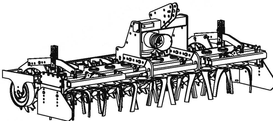
Рисунок В.1 — Роторная борона
