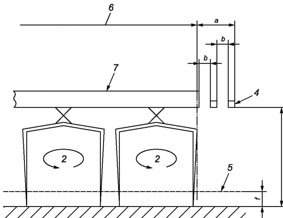
б) Боковые барьеры (см. 4.3.1)
