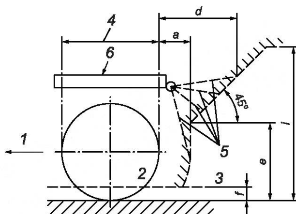
Рисунок 3 — Боковое защитное устройство (см. 4.3.1.3)
