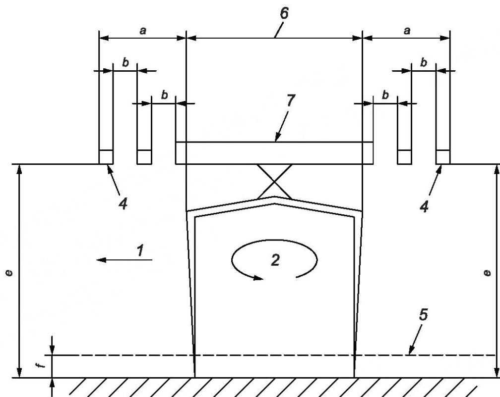
а) Передние и задние барьеры (см. 4.3.1)
