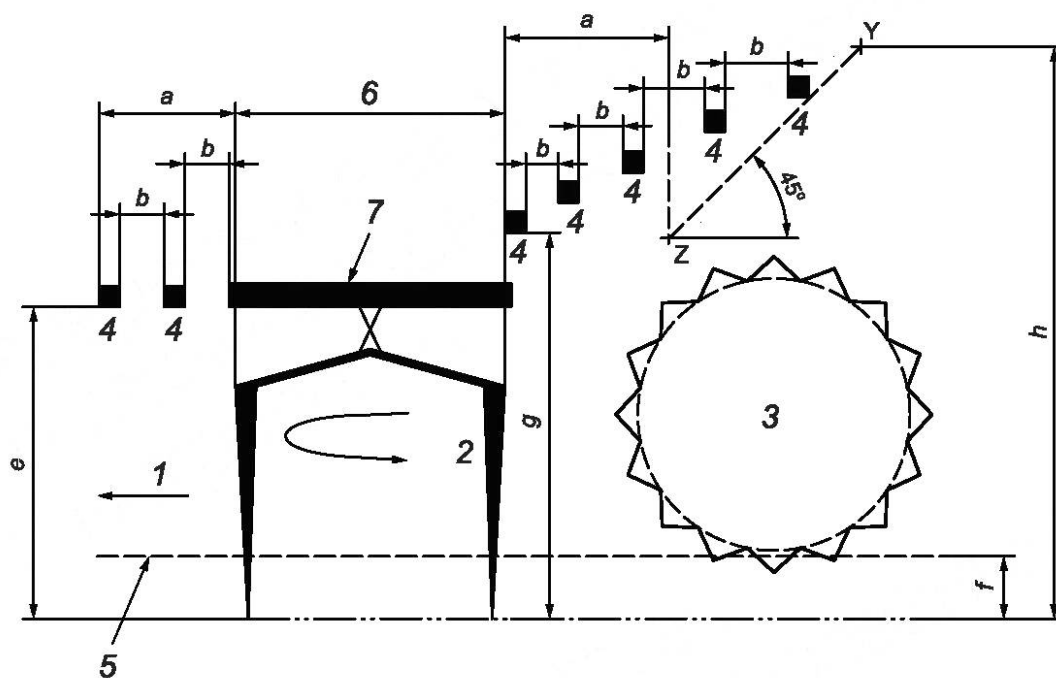
д) Заднее защитное устройство (см. 4.3.2 b), второе перечисление)
