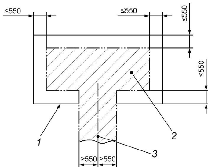
1 — внешние границы машины; 2 — недопустимая зона расположения ручных органов управления; 3 — линия симметрии машины
