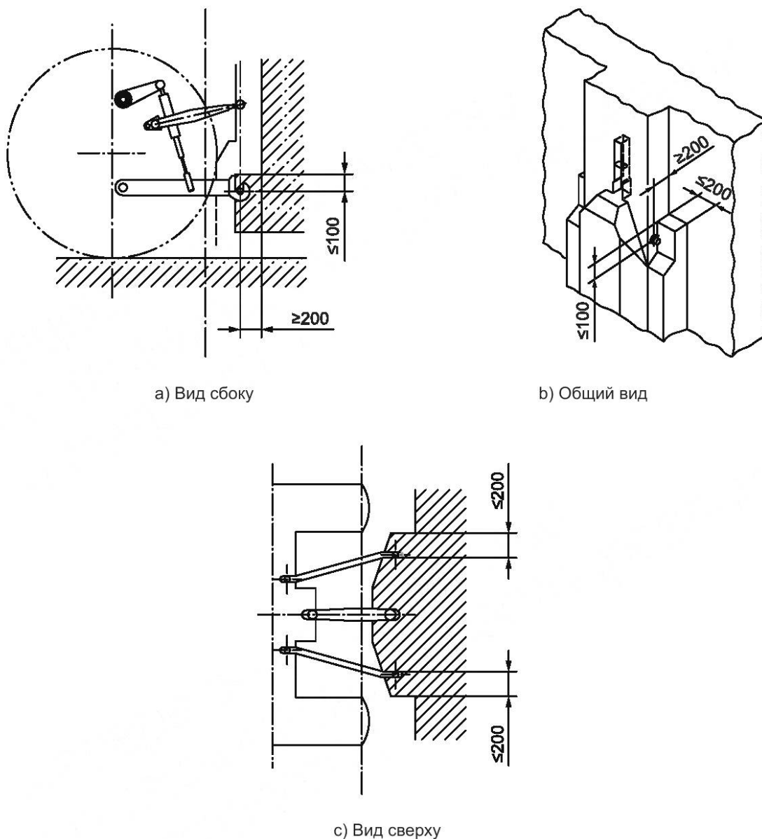
Рисунок 6 — Зона свободного пространства
