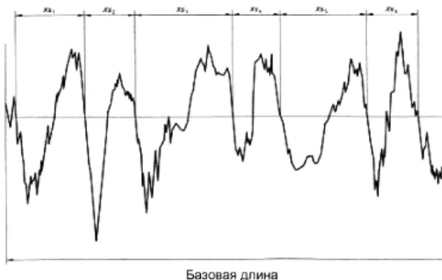
Рисунок 10 — Ширина элементов профиля
