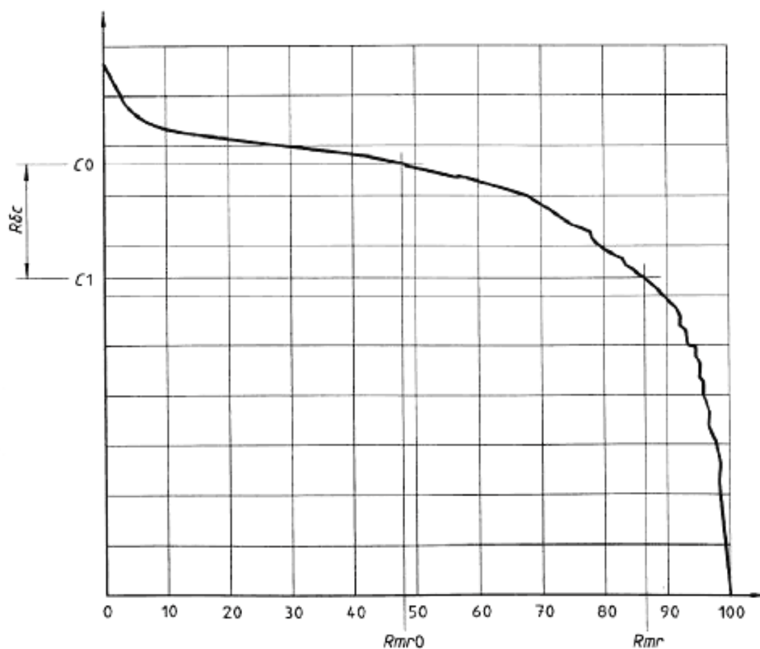
Рисунок 12 — Разделение уровня среза профиля
