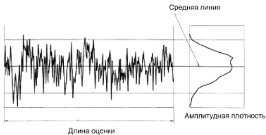
Рисунок 13 — Кривая распределения амплитуд высоты профиля
