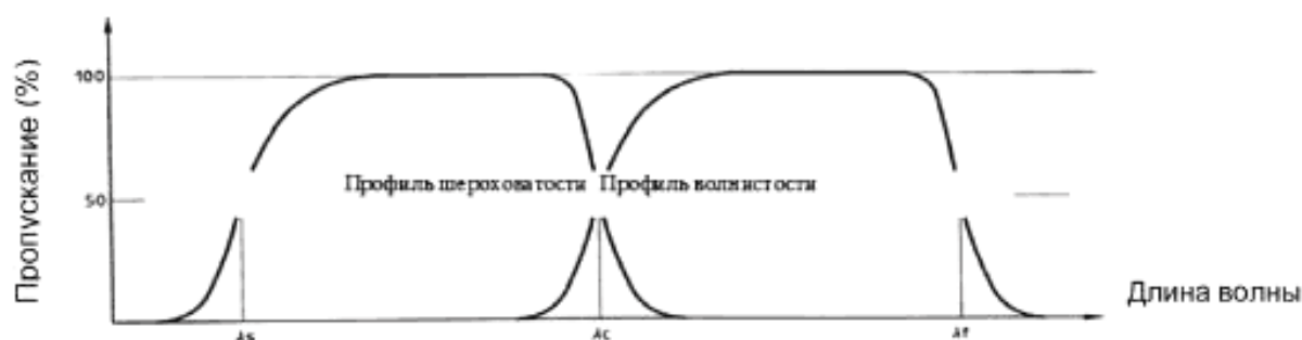
Рисунок 1 — Характеристики передачи профилей шероховатости и волнистости
