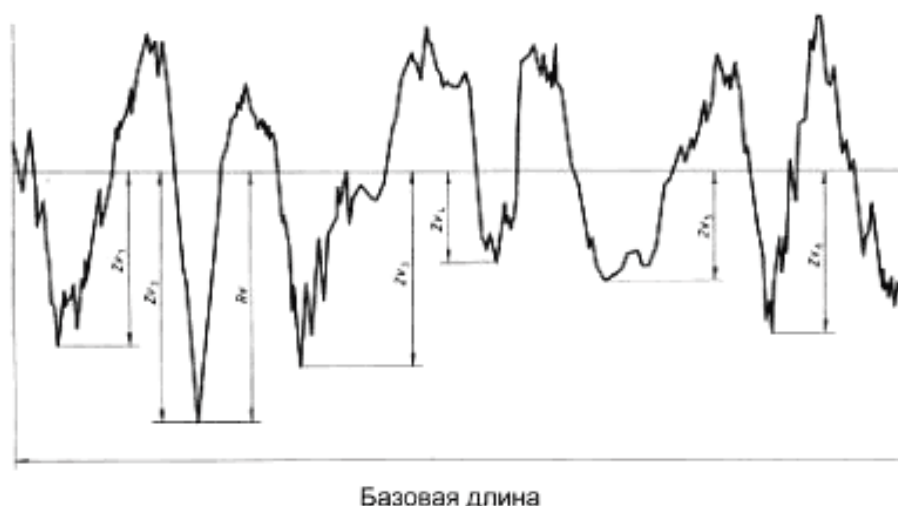
Рисунок 7 — Наибольшая глубина впадины профиля (пример профиля шероховатости)
