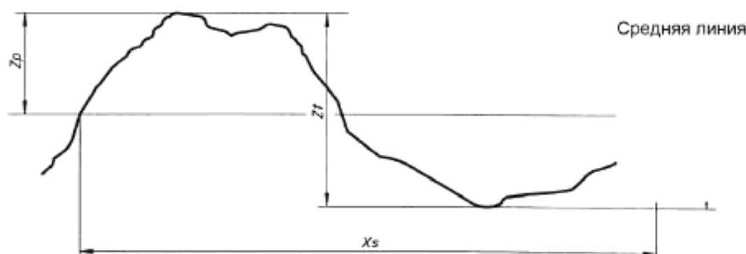
Рисунок 3 — Элемент профиля
