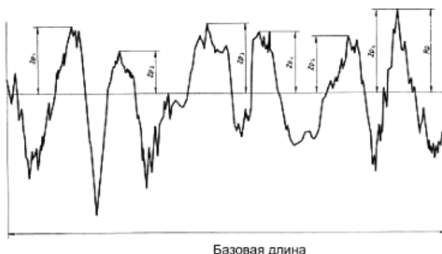
Рисунок 6 — Максимальная высота пика профиля (пример профиля шероховатости)
