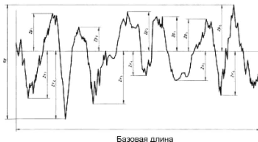
Рисунок 8 — Максимальная высота профиля (пример профиля шероховатости)
