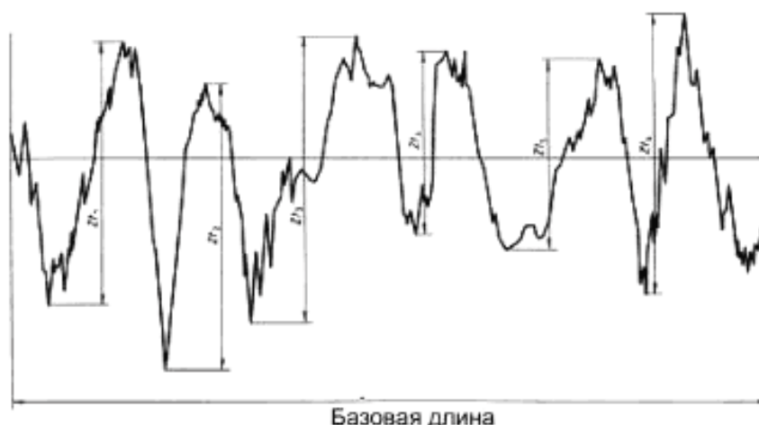
Рисунок 9 — Высота элементов профиля (пример профиля шероховатости)
