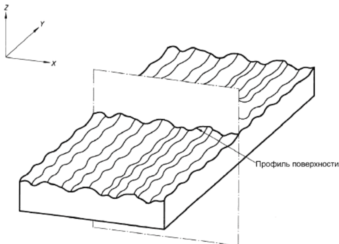
Рисунок 2 — Профиль поверхности
