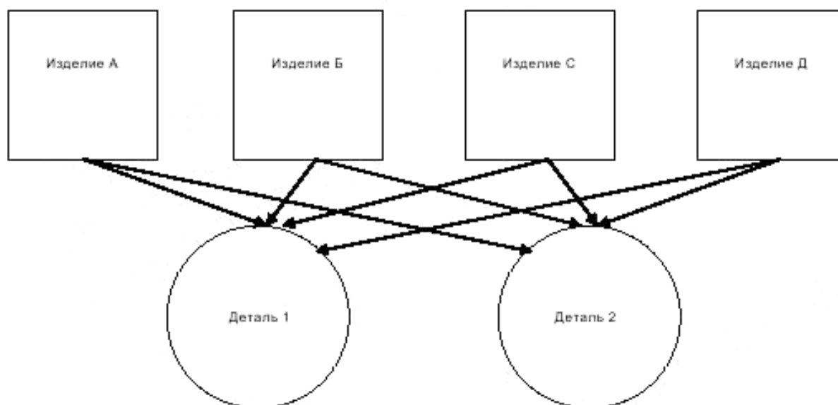
Рисунок Г.1 — Модель сетевой БД (вариант)
