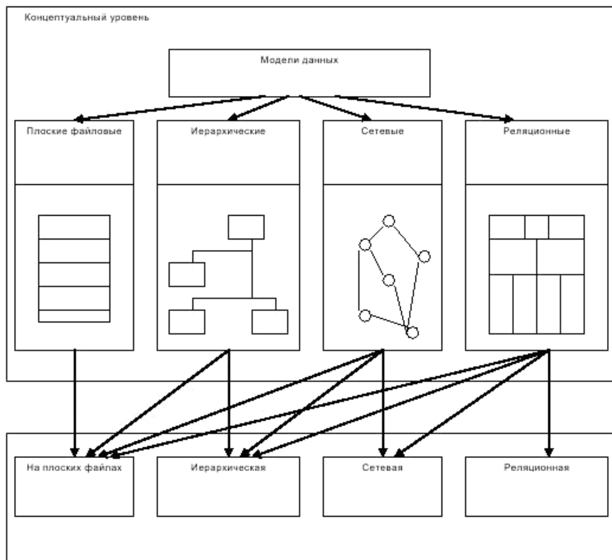
Р и с у н о к В.1 — Схема отображения моделей данных основными типами СУБД
