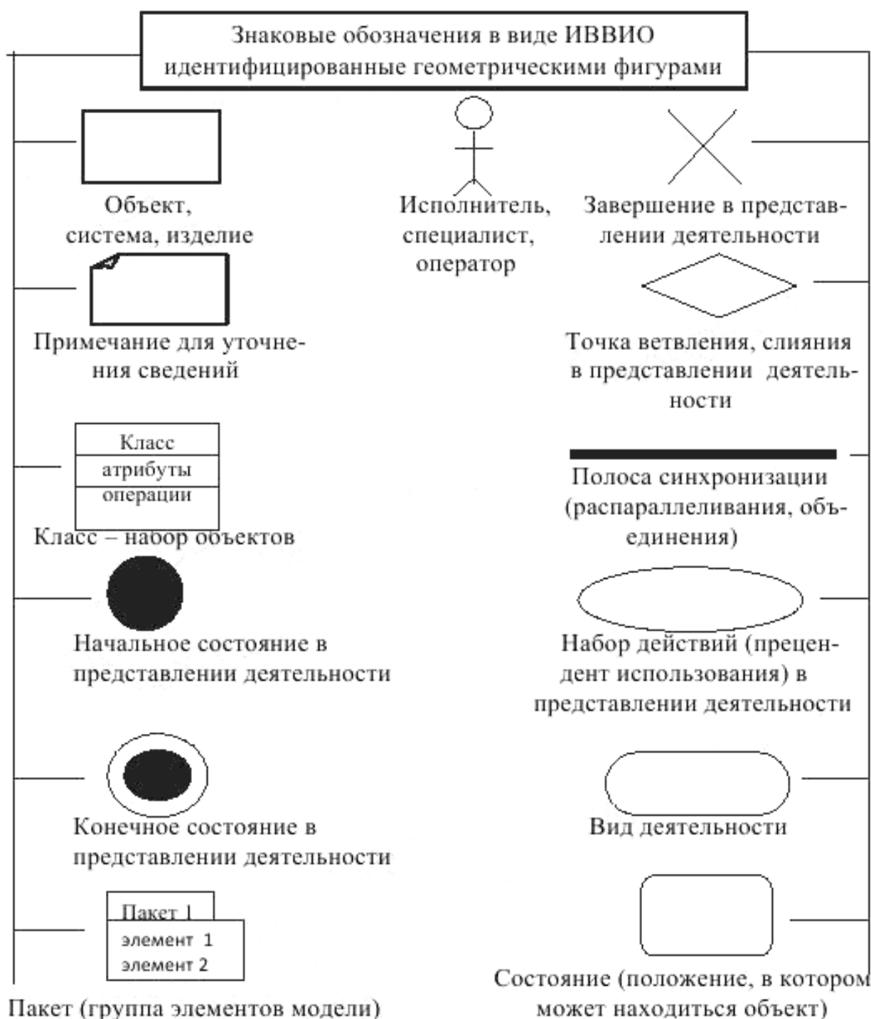
Рисунок И.1 – Примеры представления знаковых обозначений в виде ИВВИО для проведения визуального проектирования программного обеспечения
