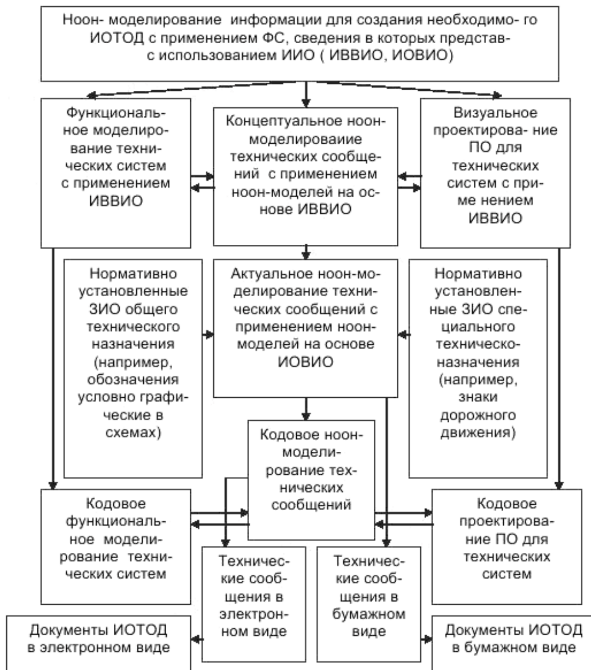
Рисунок Г.1– Схема проведения ноон- моделирования информации для создания необходимого ИОТОД с применением ФС, сведения в которых представлены с использованием ИИО (ИВВИО, ИОВИО)
