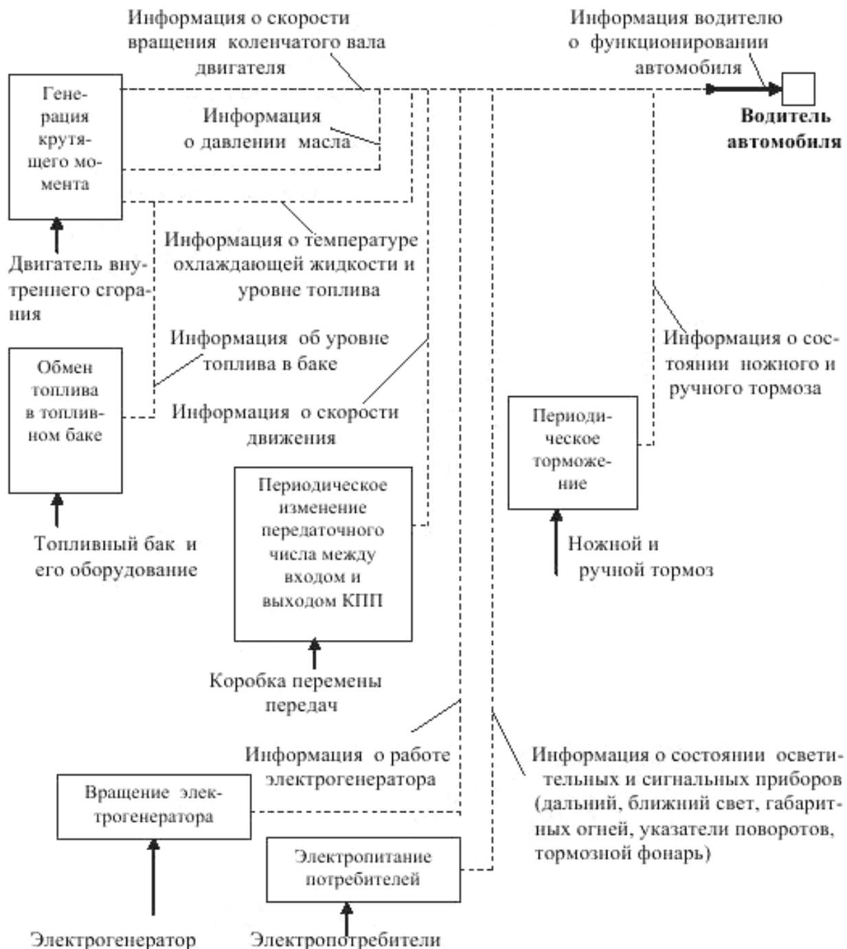
Рисунок Ж.1 – Представление в функциональном моделировании схемы функционирования информационной системы автомобиля с применением структурированных ТС в виде ИВВИО
