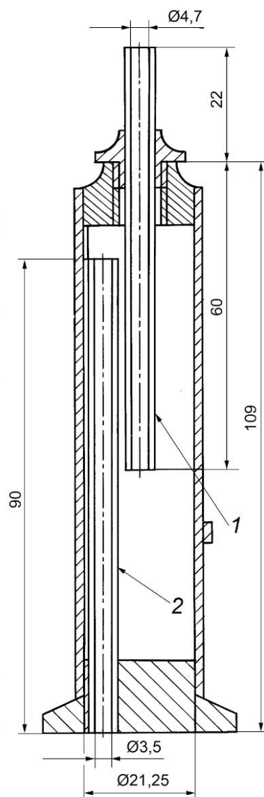
Рисунок 2 — Резервуар
