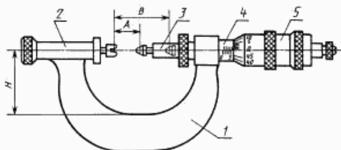
Микрометры типов МВМ, МВТ, МВП
