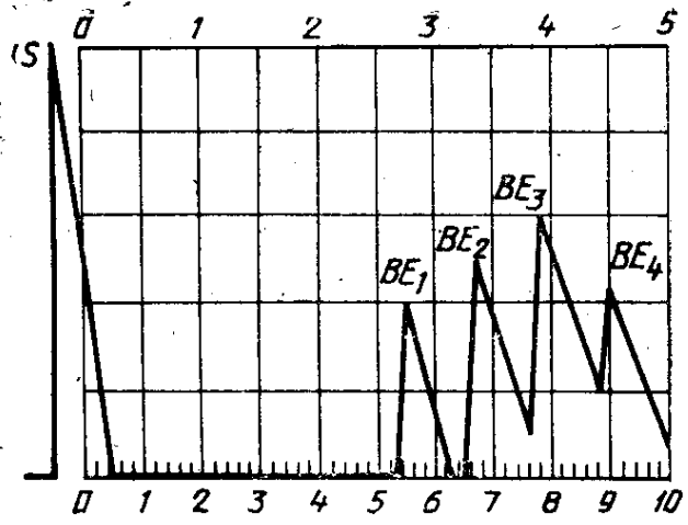
Удовлетворительное соединение (преобразователь с двумя кристаллами)
