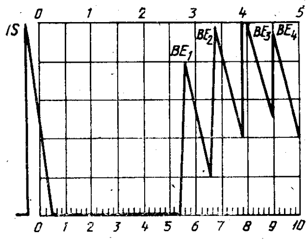
Плохое соединение (преобразователь с двумя кристаллами)
