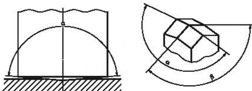
Рисунок 1 — Принцип измерения и геометрия наконечника (индентера)
