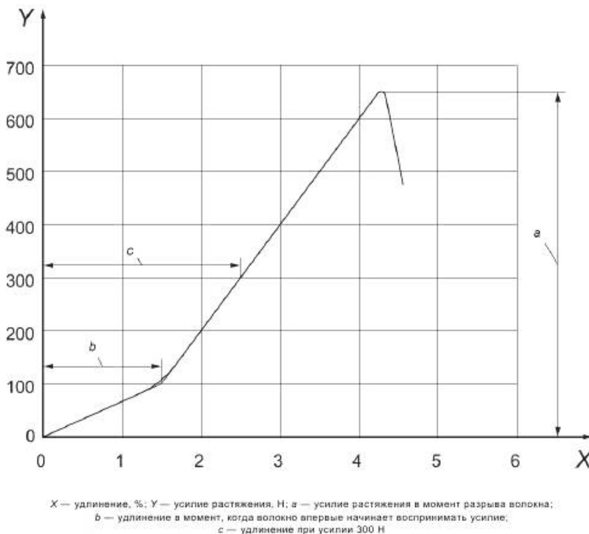
Рисунок 1 — Пример кривой усилие/удлинение
