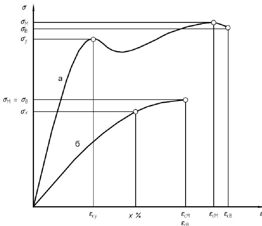
Рисунок 1 — Типичные кривые «напряжение/относительная деформация»
