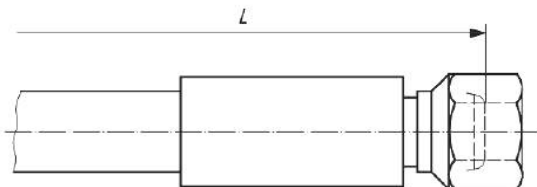
Рисунок 5 — Длина рукава между обжимными муфтами
