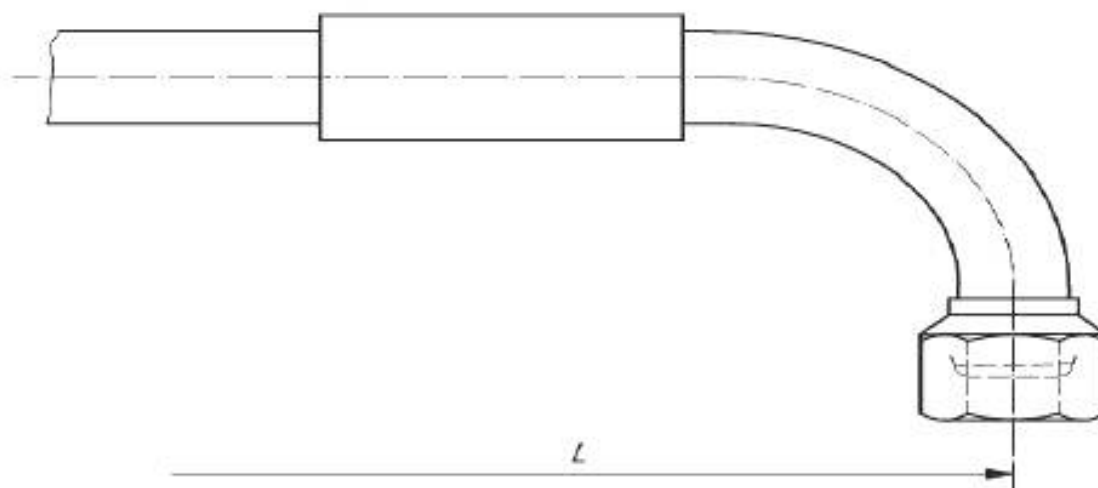
Рисунок 6 — Длина до ниппеля для присоединения рукава
