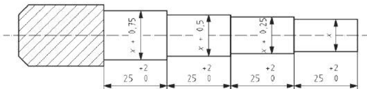
Рисунок 1 — Калибры-пробки
