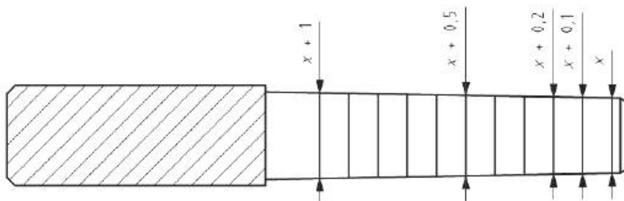
Рисунок 2 — Конусные калибры
