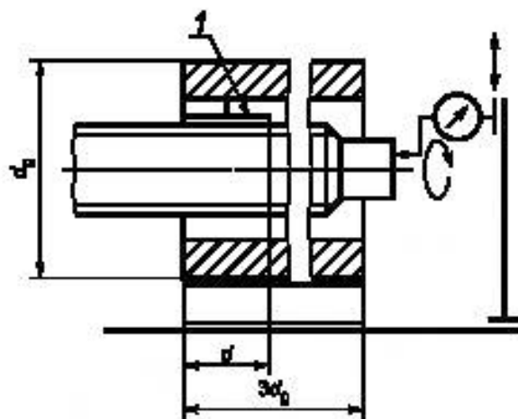
1 — трехкулачковый патрон
