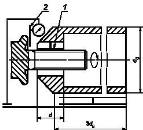
1 — трехкулачковый патрон; 2 — кромка измерительной линейки
