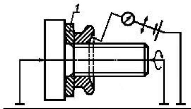
1 — коническая пружинная шайба калибра
