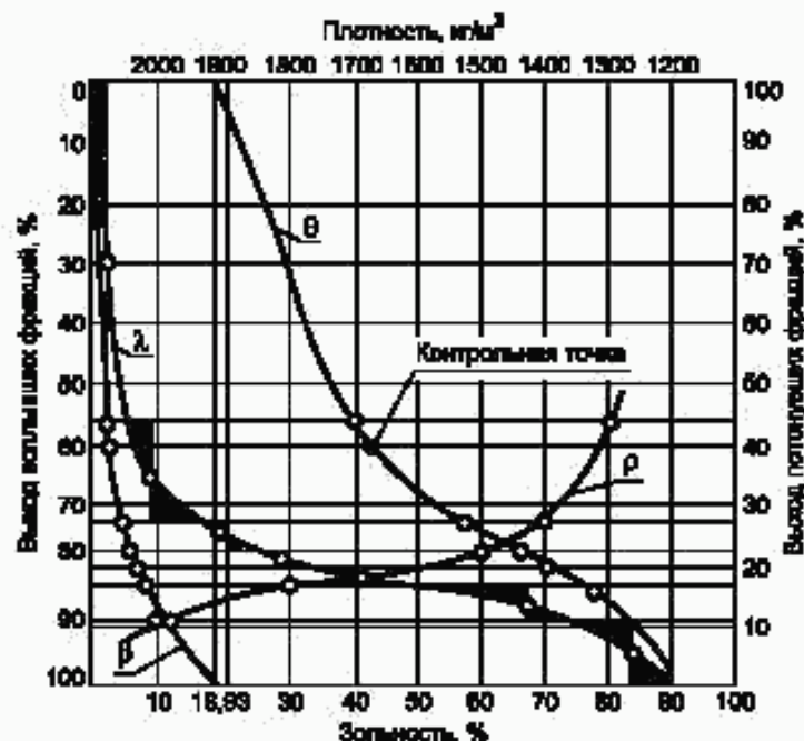
Рисунок В.1 — Кривые обогатимости
