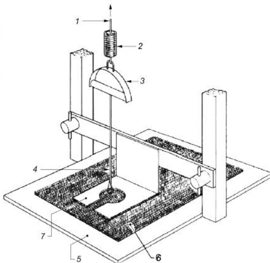
1 — нагружающий механизм; 2 — пружина (если необходимо); 3 — верхний захват; 4 — захват для пучка или крючок для петли; 5 — опорная пластина; 6 — образец ковра; 7 — зажим для образца, размеры по 5.1
