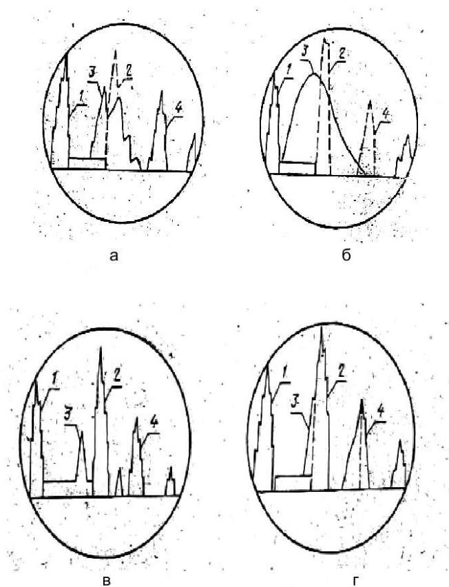
Рисунок В.1— Вид эхо-сигналов на экране дефектоскопа
