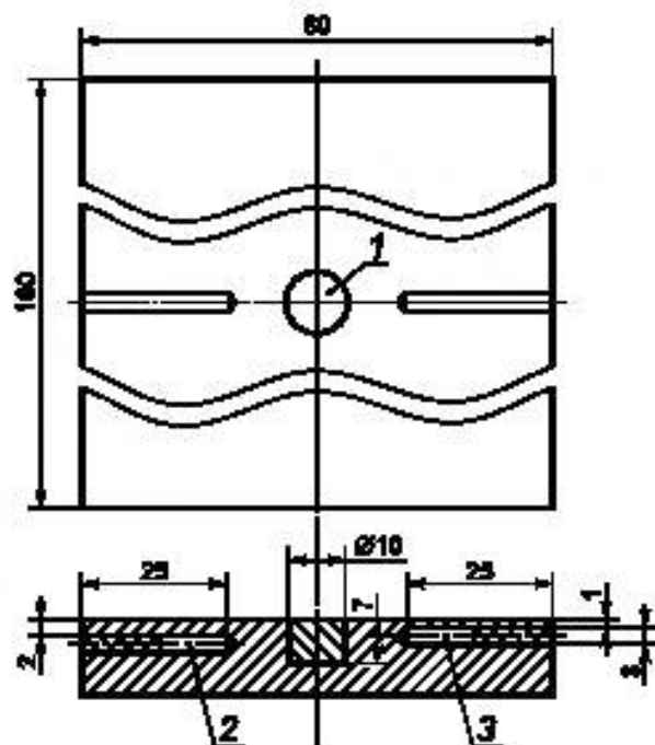
Рисунок Б.1 — Образец МО-1
