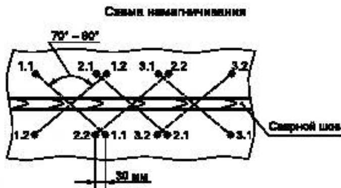
Рисунок 1 — Схема намагничивания контролируемого элемента
