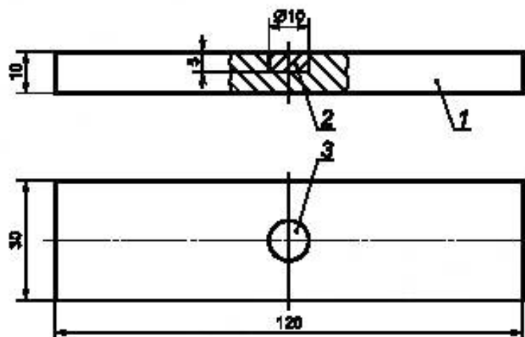
Рисунок Б.2 — Образец МО-2
