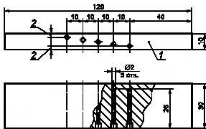
1 — брусок; 2 — цилиндрическое отверстие, закрытое винтом М 2,5
