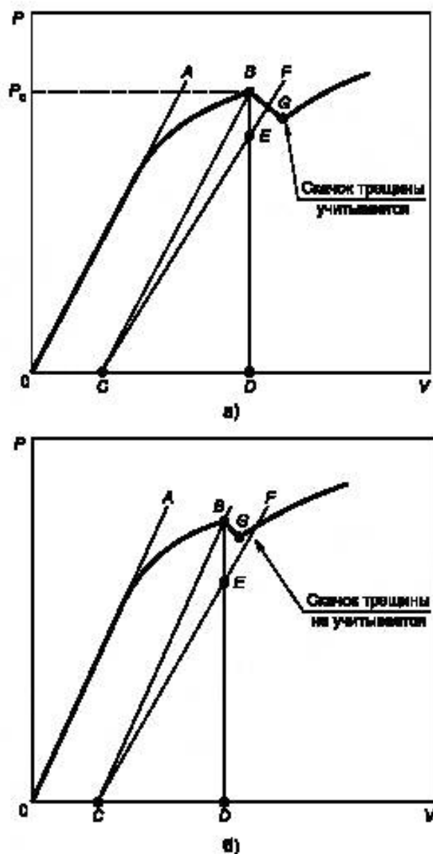
Рисунок Е.7 — Процедура оценки значимости скачка трещины
