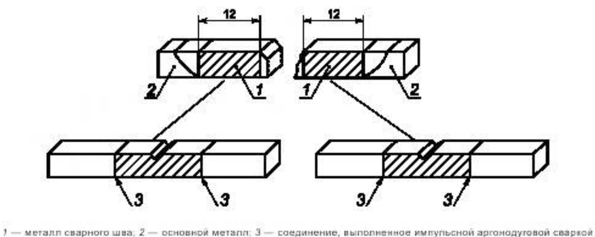
а) Реконструкция образца сварного шва
