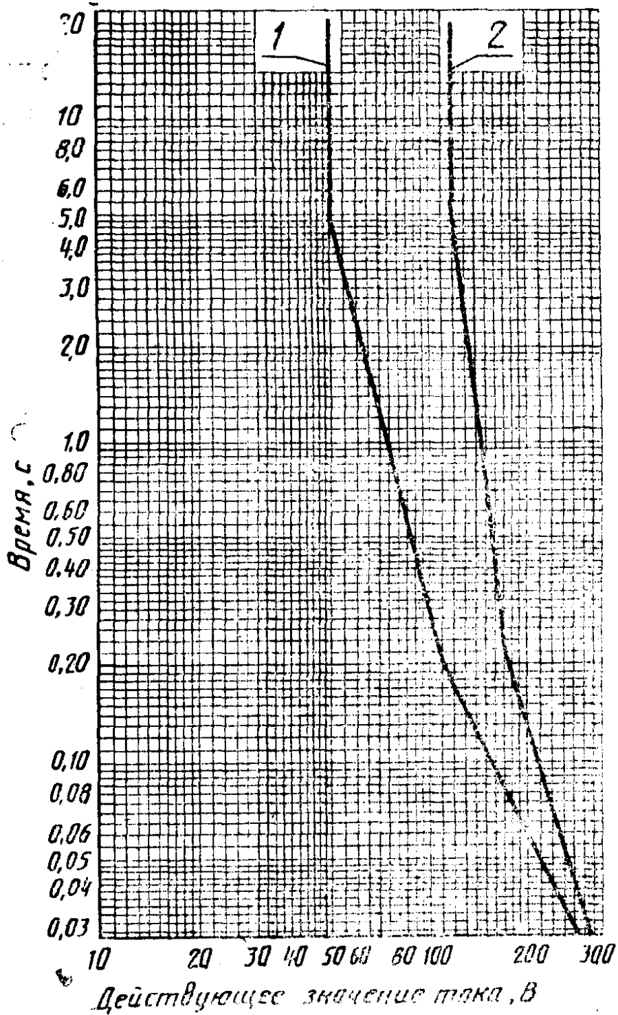
Кривая продолжительности предполагаемого напряжения прикосновения в соответствии с табл. 1
