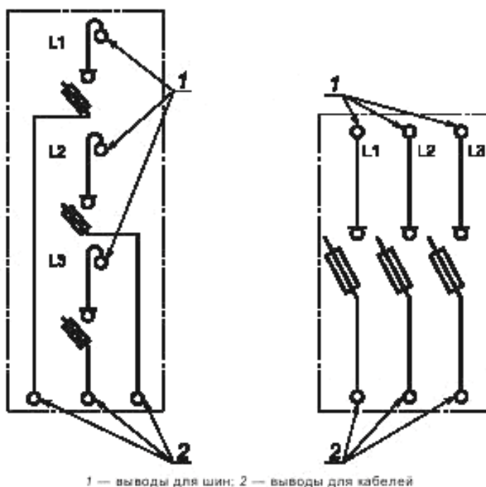
1 — выводы для шин; 2 — выводы для кабелей С.1 а) вертикальное расположение С.1 б) горизонтальное расположение
