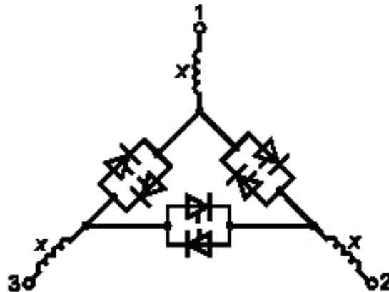
Рисунок 2b — Двигатель со схемой звезда, тиристоры со схемой треугольник;
