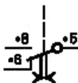
Переключающий контакт с замедлением в обеих направлениях
