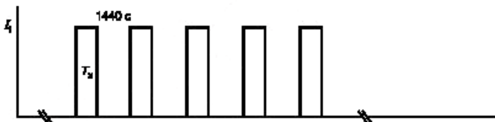
Рисунок F.1 — Профиль испытания на тепловую стабильность
