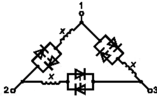
Рисунок 2а — Двигатель со схемой треугольник, тиристоры последовательно с обмоткой
