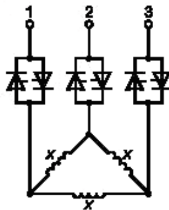
Рисунок 2с — Двигатель со схемой треугольник, тиристоры соединены между обмоткой и источником питания.
