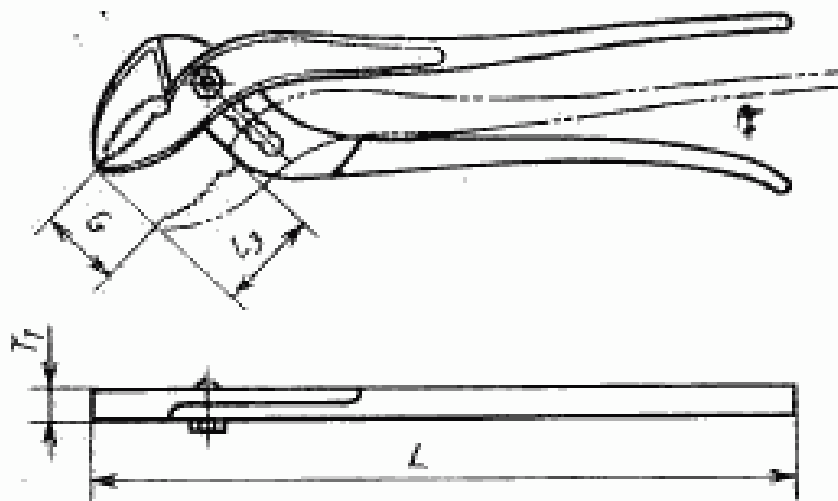
Исполнение 1
