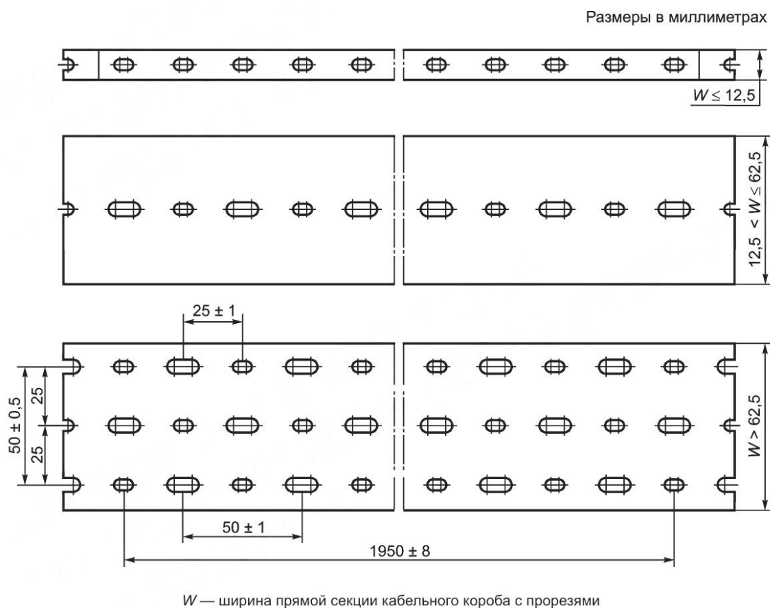
Рисунок 101 — Примеры схем крепления отверстий в основании прямой секции кабельного короба с прорезями
