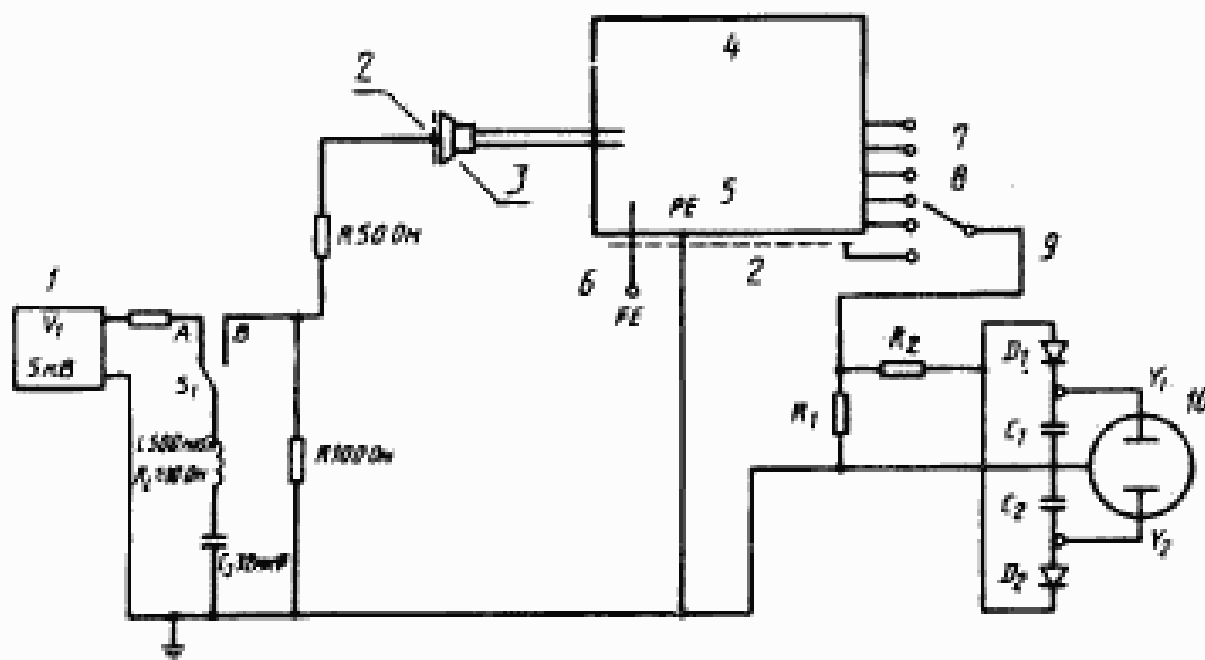
1 — источник постоянного напряжения 5 кВ; 2 — ПРЕОБРАЗОВАТЕЛЬ; 3 — металлическая фольга; 4 — испытуемый прибор; 5 — ЗАЖИМ ЗАЩИТНОГО ЗАЕМЛЕНИЯ (для приборов класса I); 6 — ЗАЖИМ РАБОЧЕГО ЗАЕМЛЕНИЯ; 7 — часть СИГНАЛЬНОГО ВХОДА; 8 — часть СИГНАЛЬНОГО ВЫХОДА; 9 — корпус прибора; 10 — дифференциальный осциллограф с погрешностью 5%, входное со- противление Z_{\text{вх}} = 1 \text{ МОм} . R_1 : 1 кОм \pm 2\% , номинальное напряжение не менее 2 кВ; R_2 : 100 кОм \pm 2\% , номинальное напряжение не ме- нее 2 кВ; C_1, C_2 : 1 мкФ \pm 5\% ; D_1, D_2 — диоды малых сигналов.
