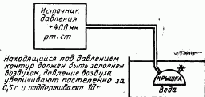
Рисунок 106 — Испытание герметичности диафрагмы (см. 17.101.2)
