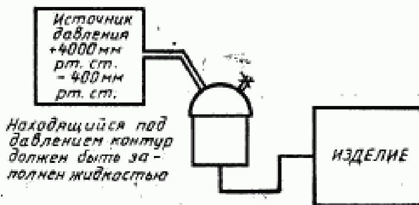
Рисунок 107 — Испытание давления, наращаемого постепенно (см. 45.101)
